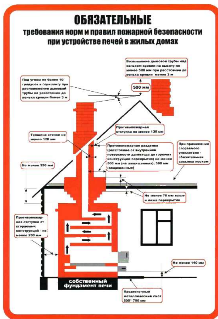
Рисунок 35. Обязательные требования норм и правил пожарной безопасности при устройстве печей в жилых домах
